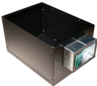
Fig. 60 1681BL-11 IC Box
