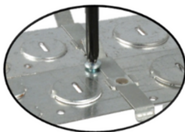
Fig. 41 Triparloc™
